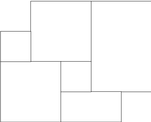
VERSAILLES PATTERN (1) 16x24, (2) 16x16, (1) 8x16, (2) 8x8, 8 SF
